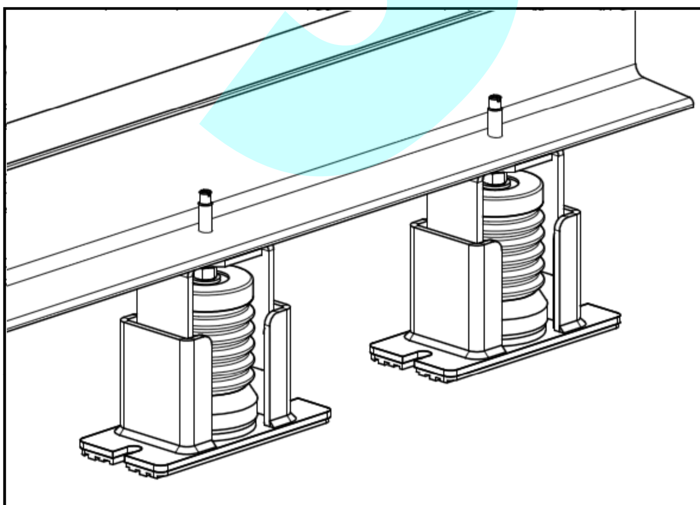
圖3)將避震器置入安裝機器之位置。
