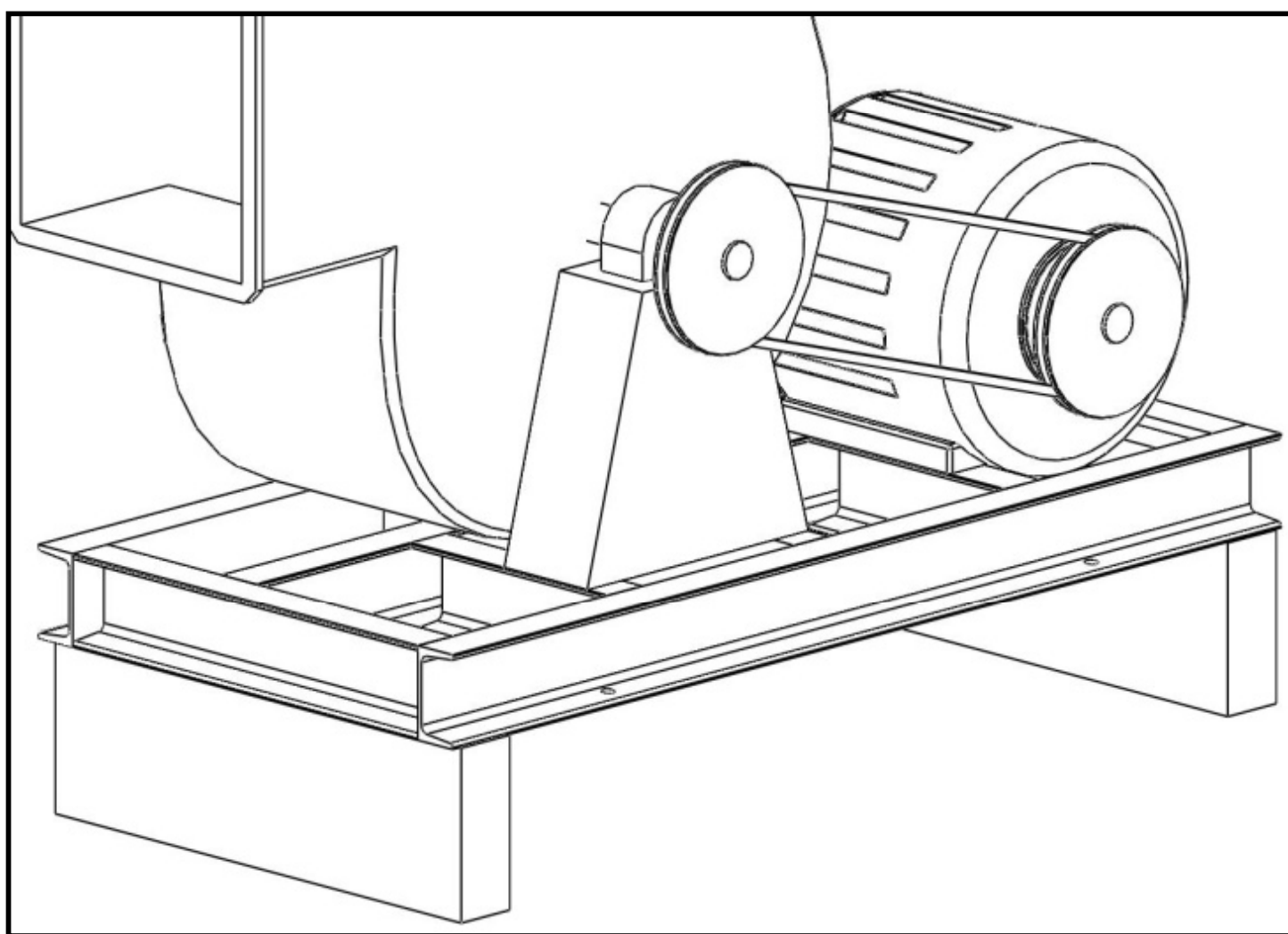
圖1)安裝設備時可先放置與避震器相同高度之臨時木台。
